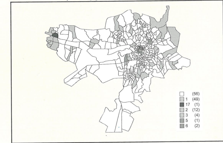
Harita-3. 1994 ve 1995 yıllarında yapılan değişikliklerin mahallelere göre dağılımı
