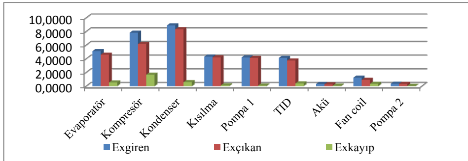
Şekil 7. Soğutma sezonu için elemanlara ait ekserji değerleri
