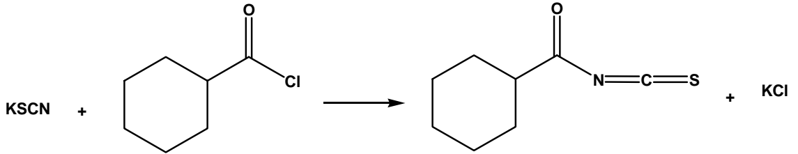
Şekil 3.1 Sikloheksankarbonilizotiyosiyanat sentezi.
