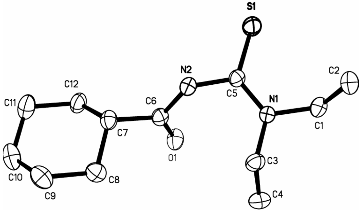
Şekil 4.1 N -(dietilkarbamotiyoil)sikloheksankarboksamid ligandının kristal yapısı.
