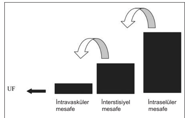
ŞEKİL 1: UF'da sıvı alım mekaniği ve yeniden dolum. 17 İntervasküler alandan çekilen sıvının yerini önce interstisyel alandan sonra da hücre içinden çıkan su doldurur.
