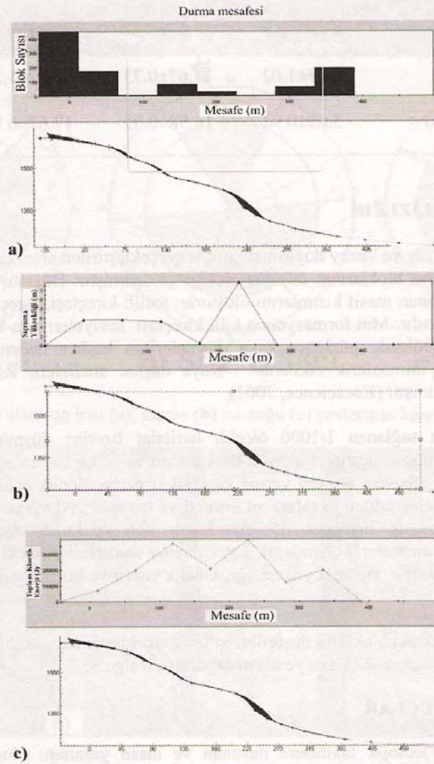
Şekil 8. X-X' hattında blokların durma mesafeleri (a), Sıçtama yüksekliği (b) ve kinetik enerjisi (c).
