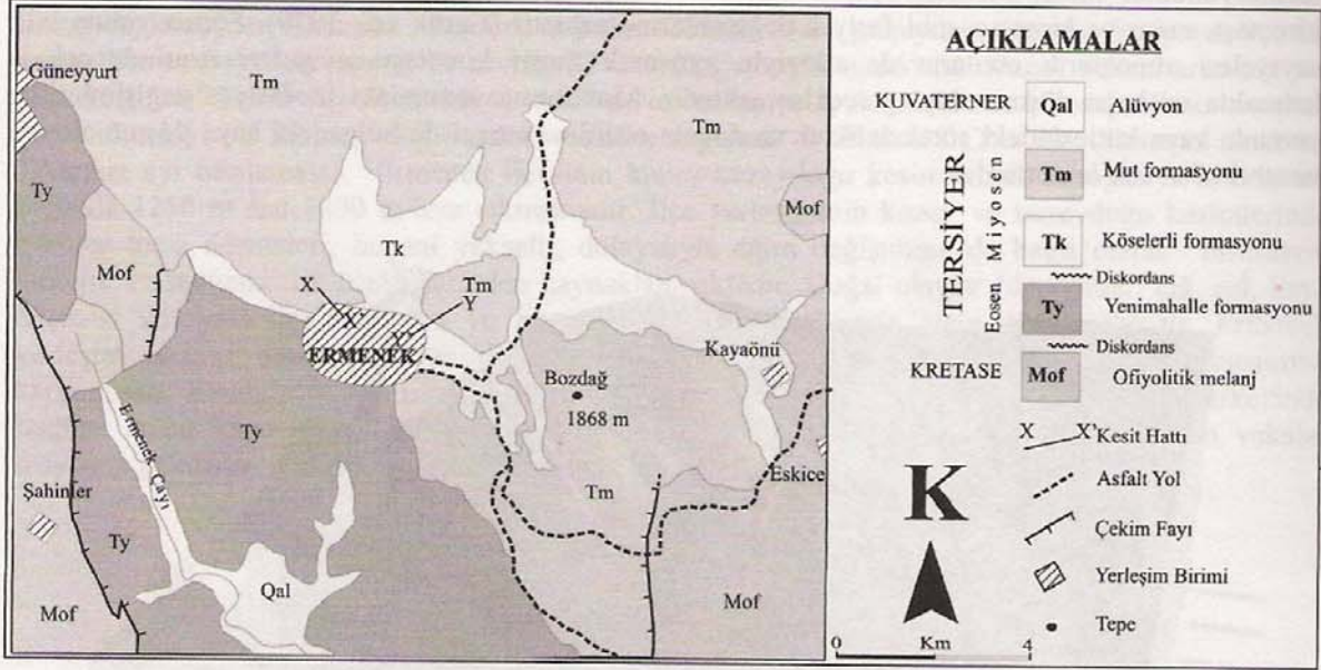
Şekil 3. Ermenek ve civarının jeoloji haritası (Gedik vd., 1979'dan yalınlaştırılarak).
