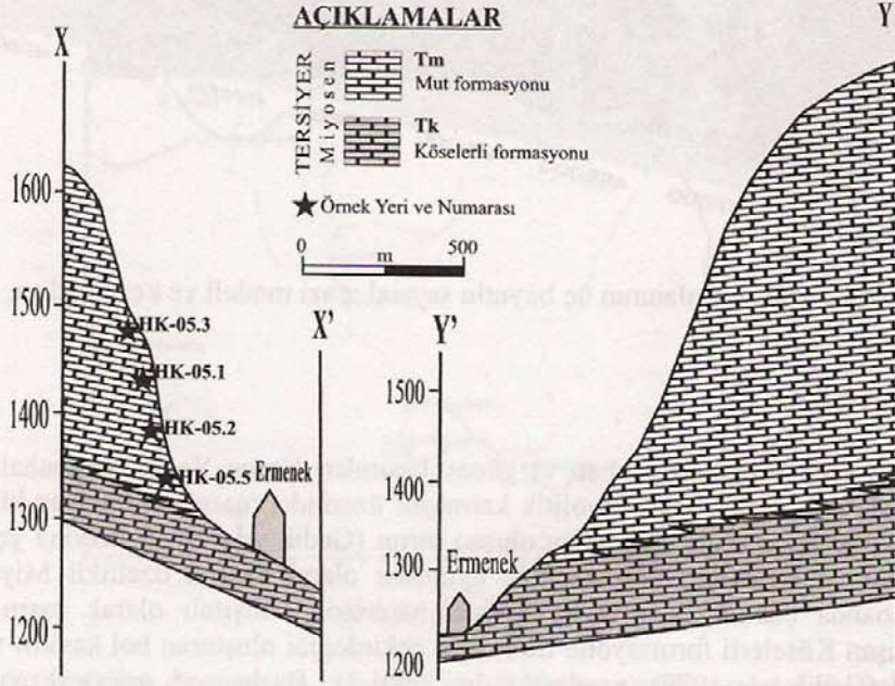
Şekil 4. X-X' ve Y-Y' hatlarından alınmış stratigrafik kesit.
