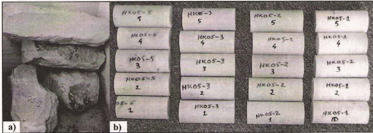
Şekil 7. İndeks ve tek eksenli sıkışma dayanımının belirlendiği örneklerden bir görünüm.
