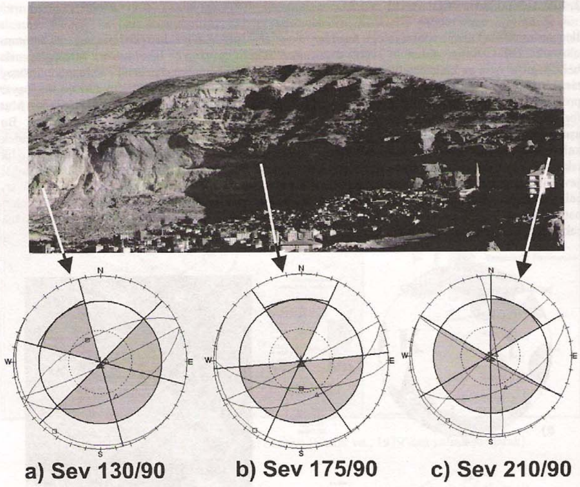
Şekil 6. İnceleme alanının batı (a), kuzey (b) ve doğu (c) şevlerinin kinematik incelemesi.
